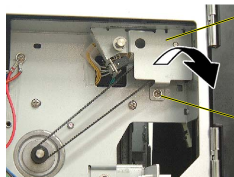
Platen Gear Frame
