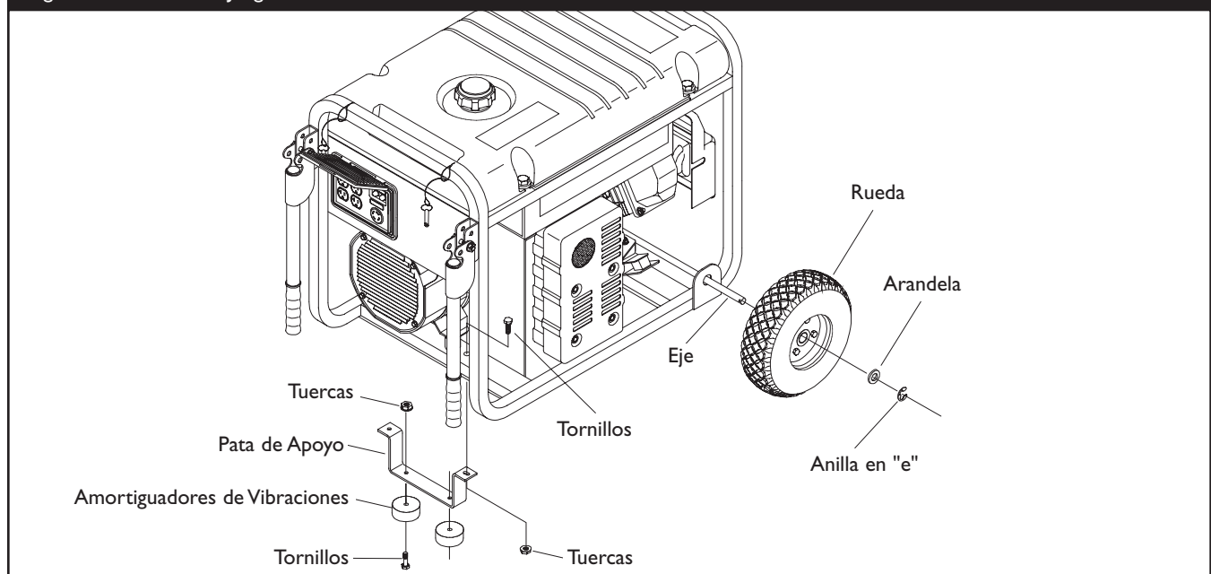
Figura 12 — Instale el Juego de Ruedas
