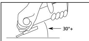
Figura 3 - Ángulo incorrecto
