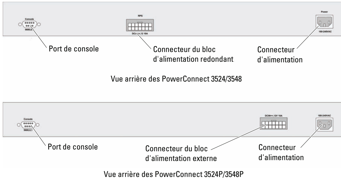
Figure 1-3. Connecteur d'alimentation du panneau arrière
