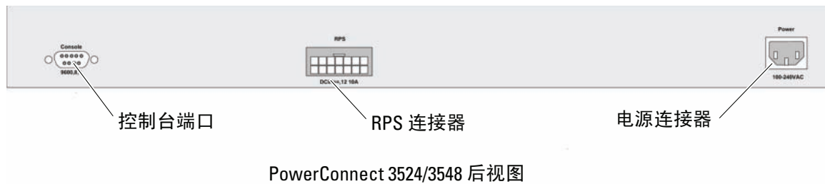
图 1-3. 背面板电源连接器
