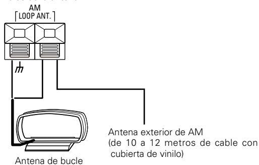
Terminales de la antena AM
