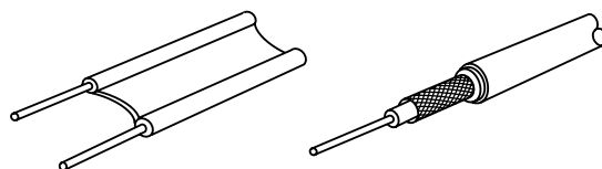
Cable de alimentación de 300 ohmios Cable coaxial de 75 ohmios
